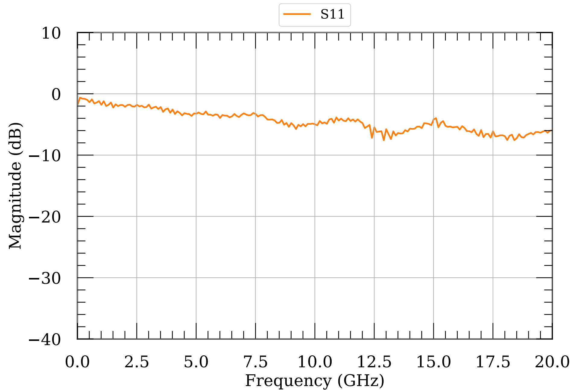
LNA S-params module084
